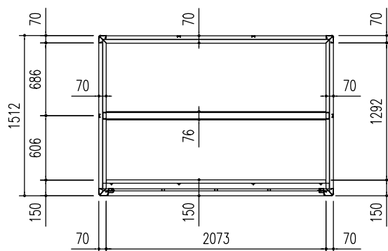
床 伏 図 (S = 1/50)
