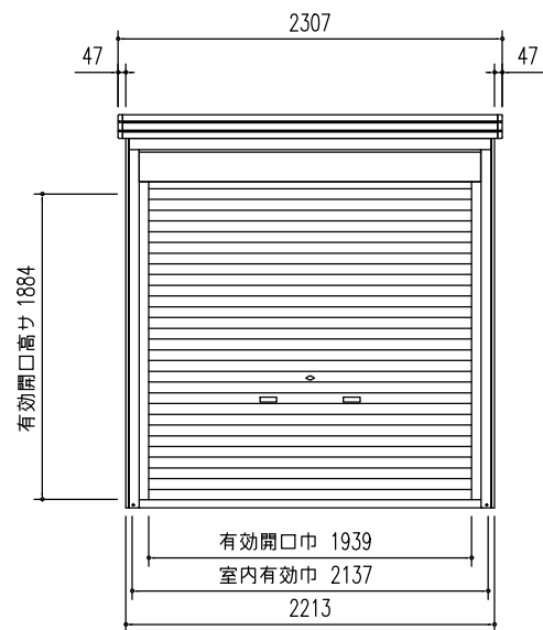
正面立面图 (S = 1/50)
