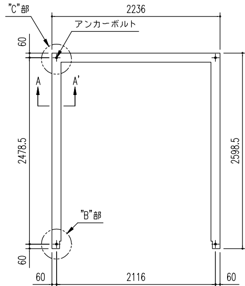
布基礎伏図 (S=1/50)
