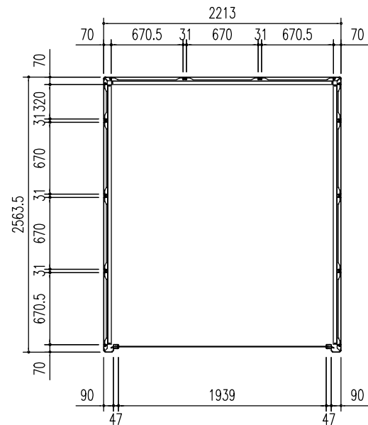
平面図 (S=1/50)
