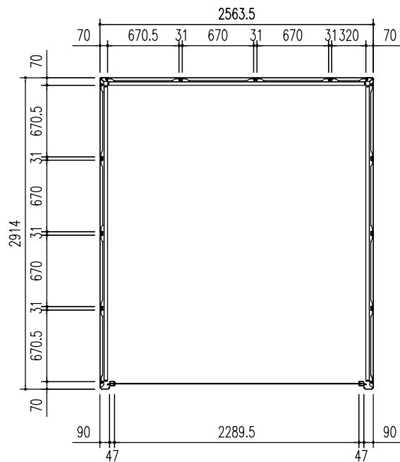
平面図 (S = 1/50)
