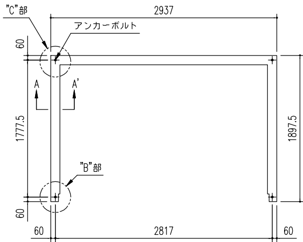
布基礎伏図 (S=1/50)
