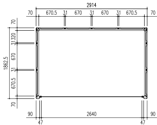
平面図 (S=1/50)
