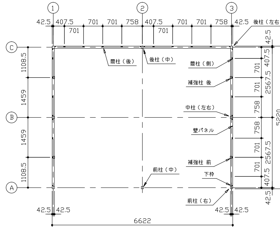
平面図 (S=1/80)
